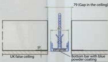
Abschlussleiste
